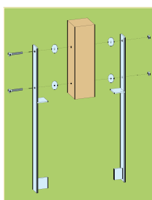
H-Pfostenanker Art.-Nr. 08743
