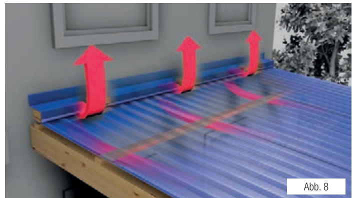
Abb. 8 Ein hinterlüfteter Wandanschluss sorgt für den nötigen Luftaustritt, damit sich die Kondensatbildung verringert.
